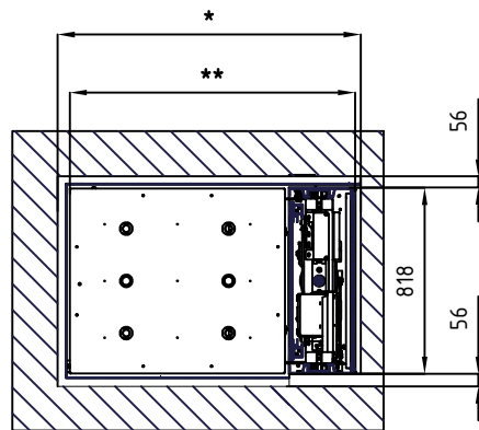
A-A
